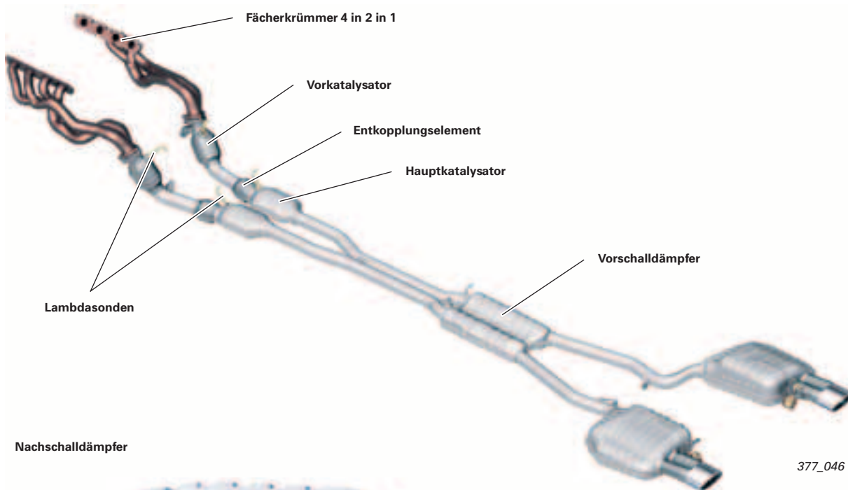
Abgasanlage RS4
