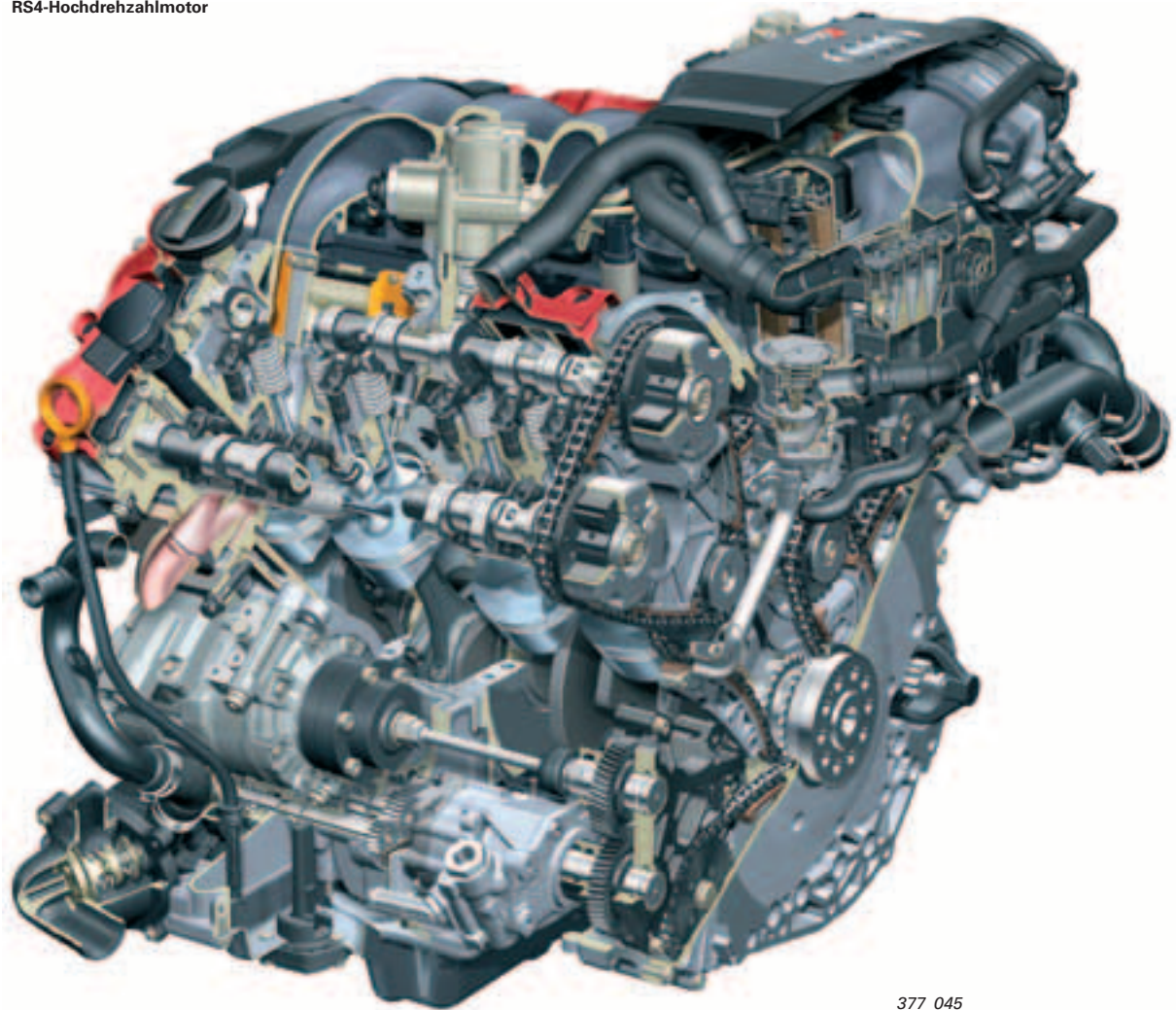
RS4-Hochdrehzahlmotor
