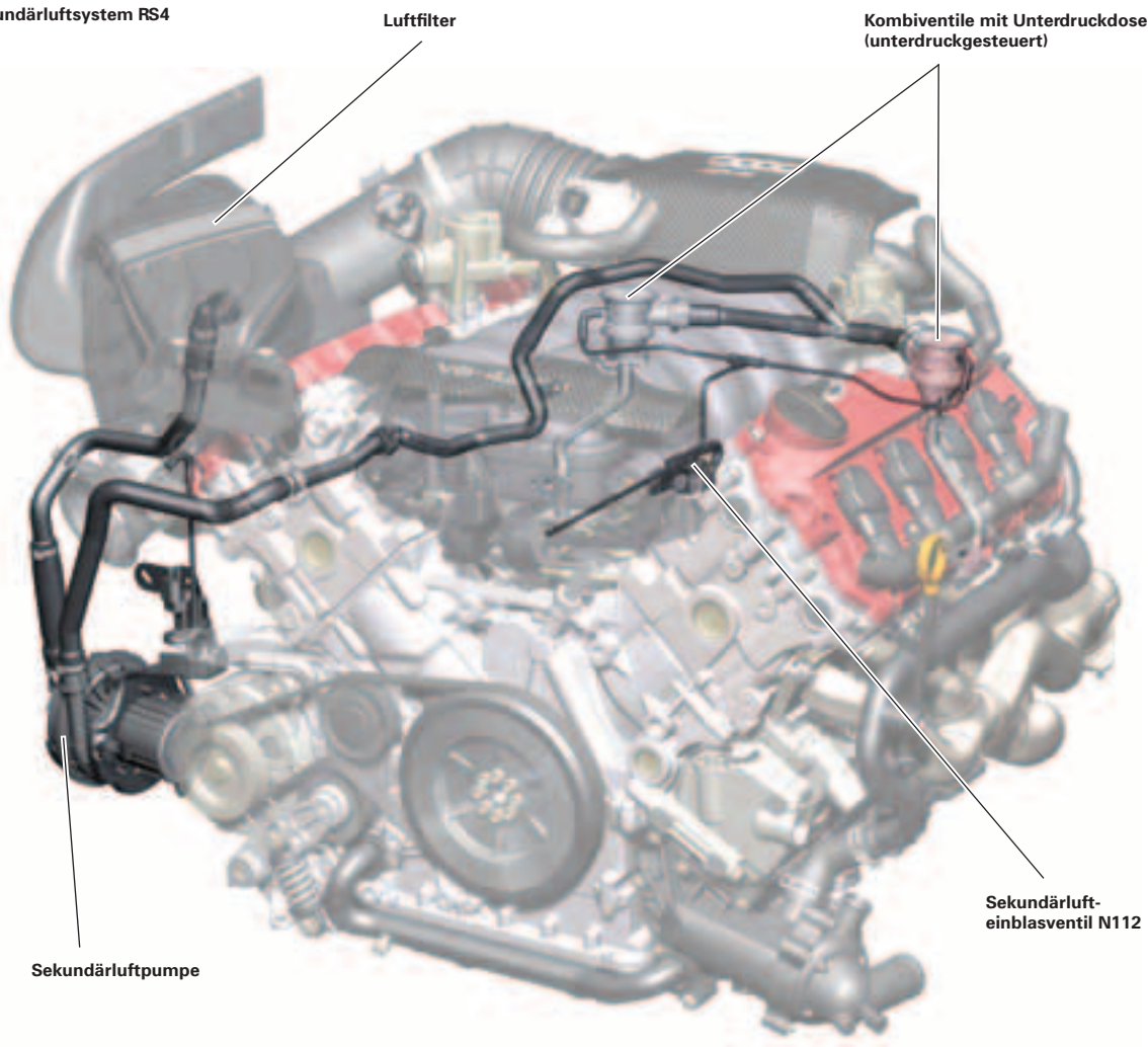
Sekundärluftsystem RS4
