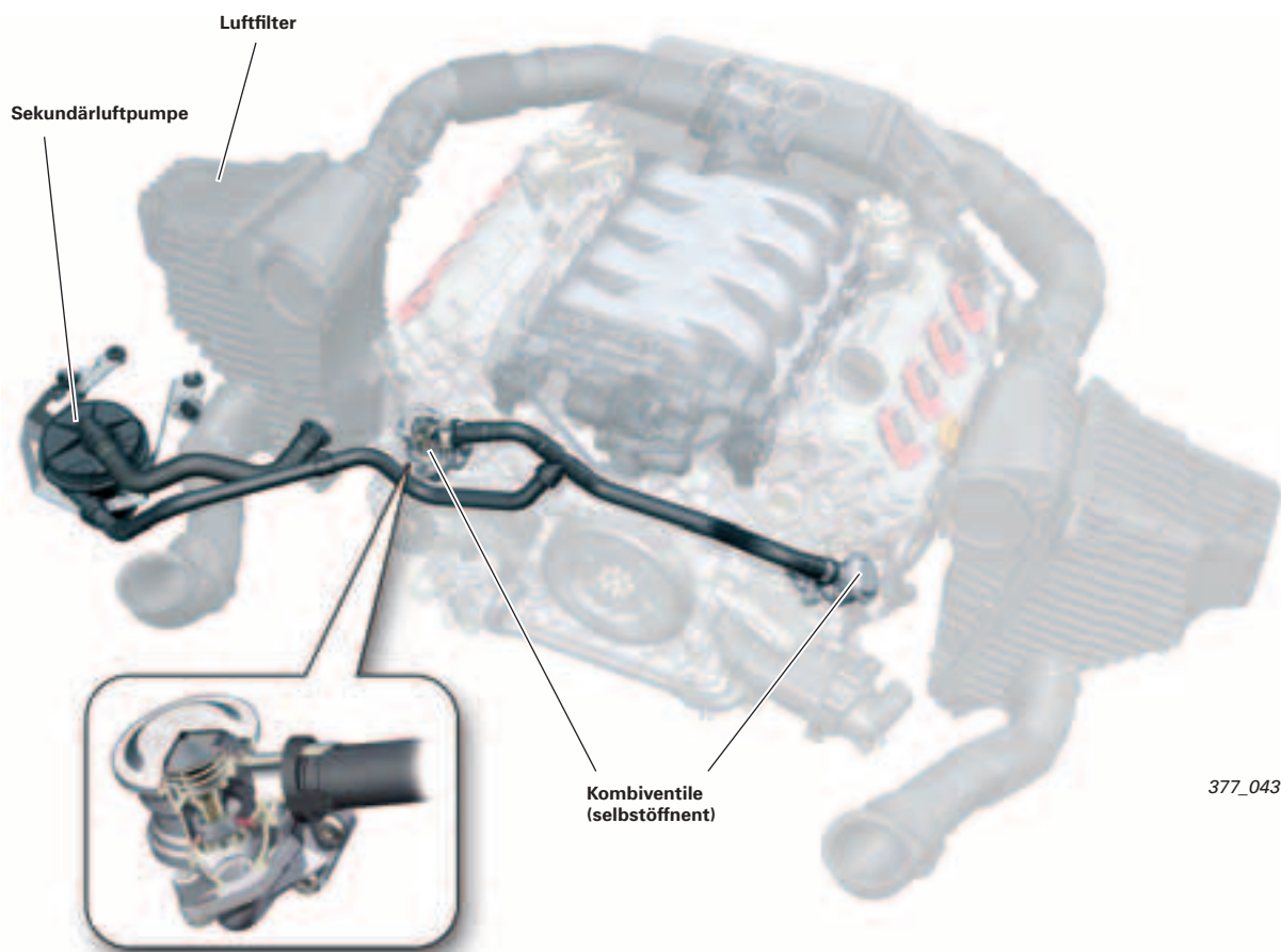
Sekundärluftsystem Q7
