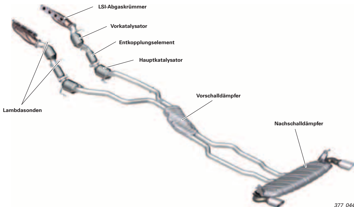
Abgasanlage Q7
