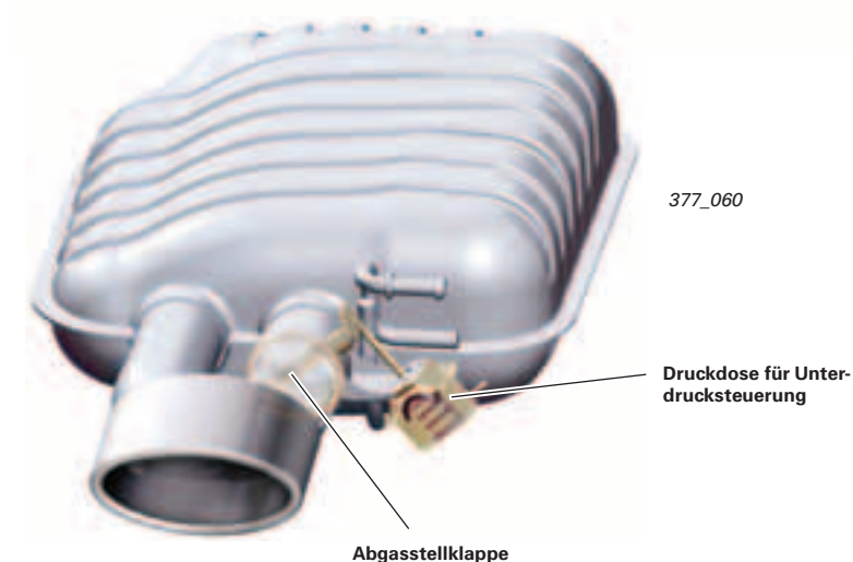
Nachschalldämpfer
